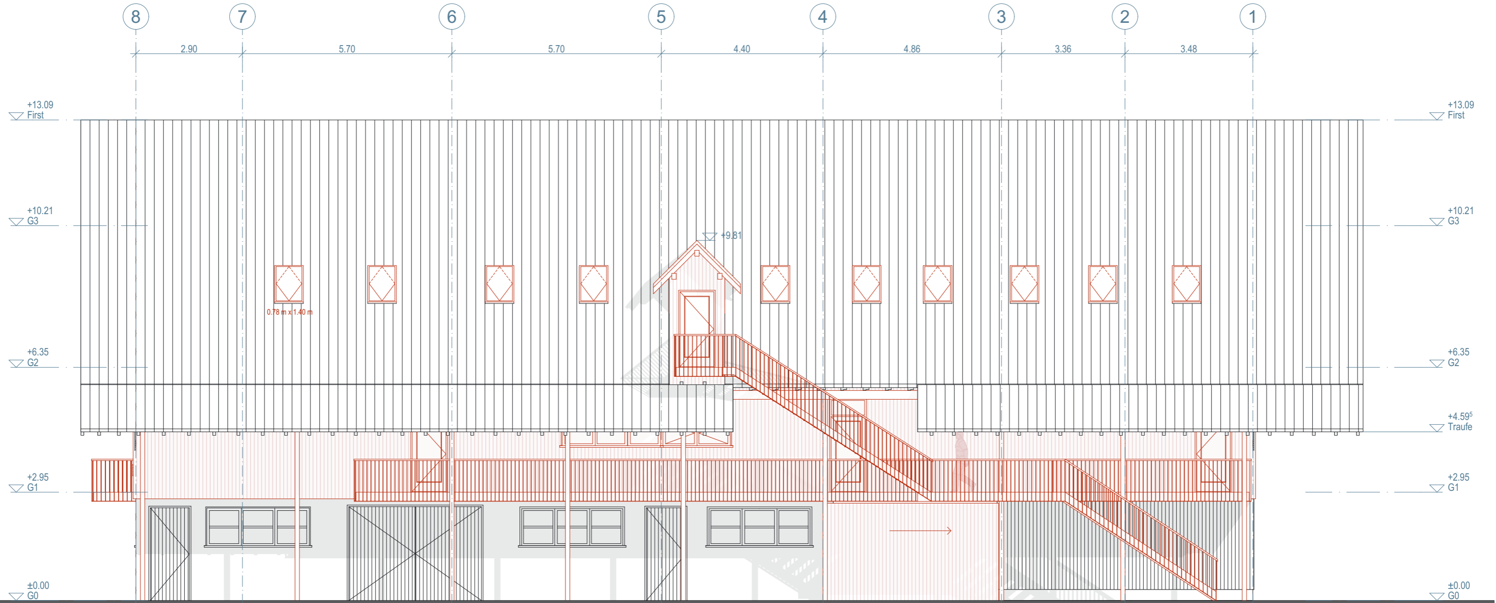
Ansicht Ost
