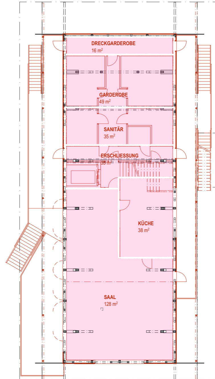
G1 Flächen Neu 1:200
