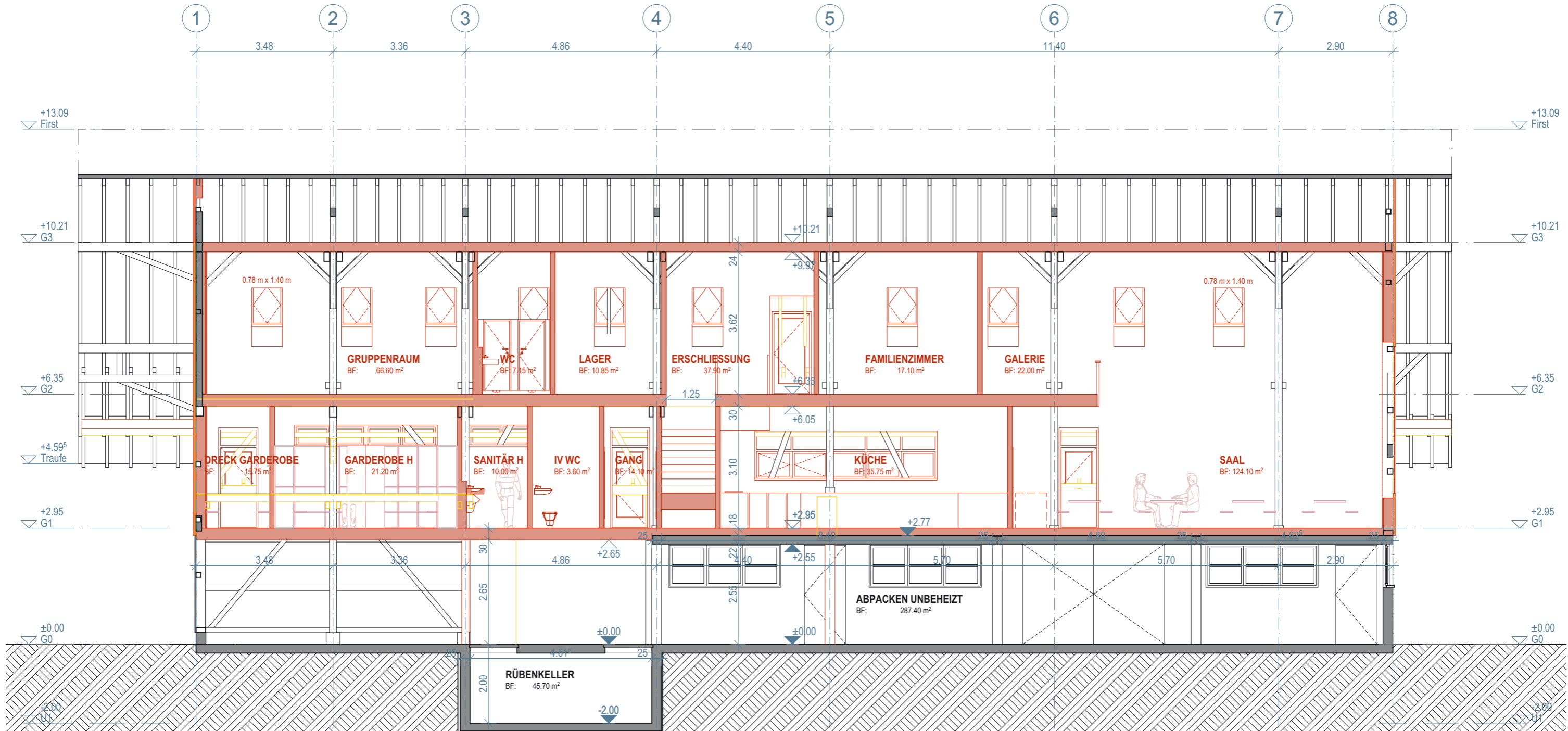
Längsschnitt S/03
