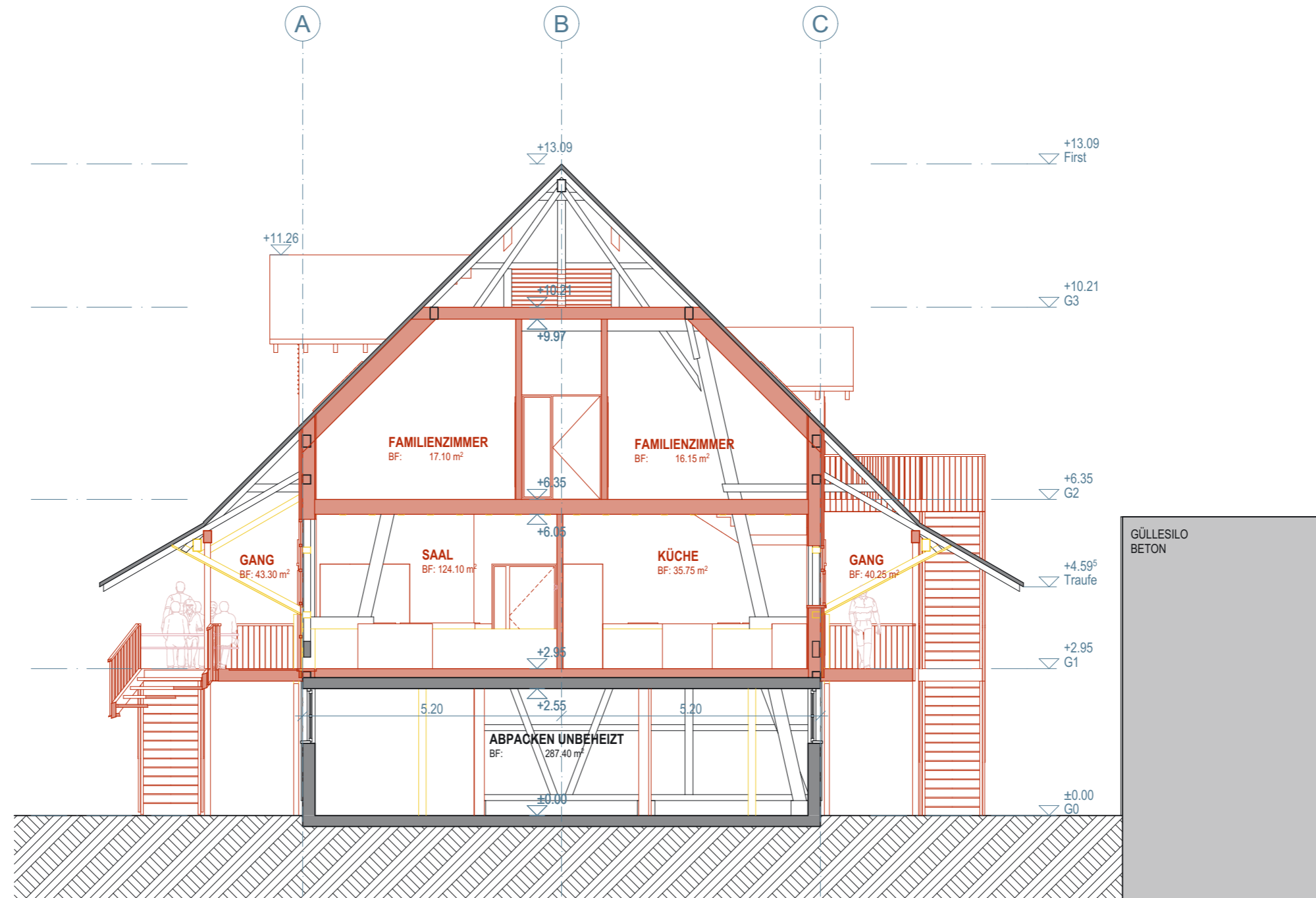
Querschnitt S/01
