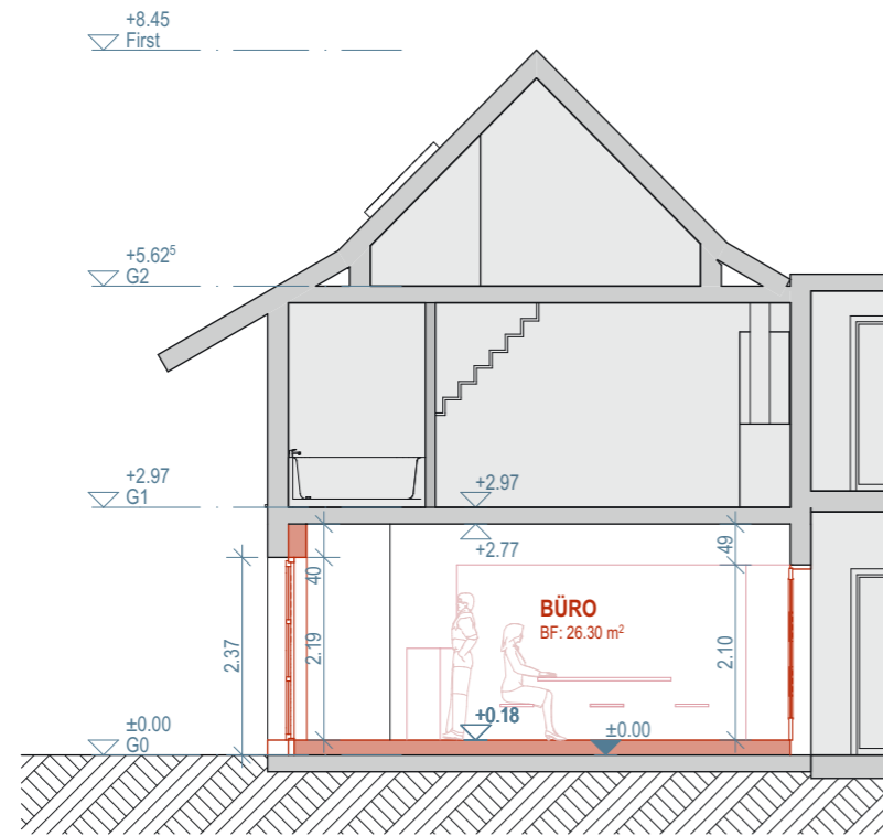
S/01 Querschnitt
