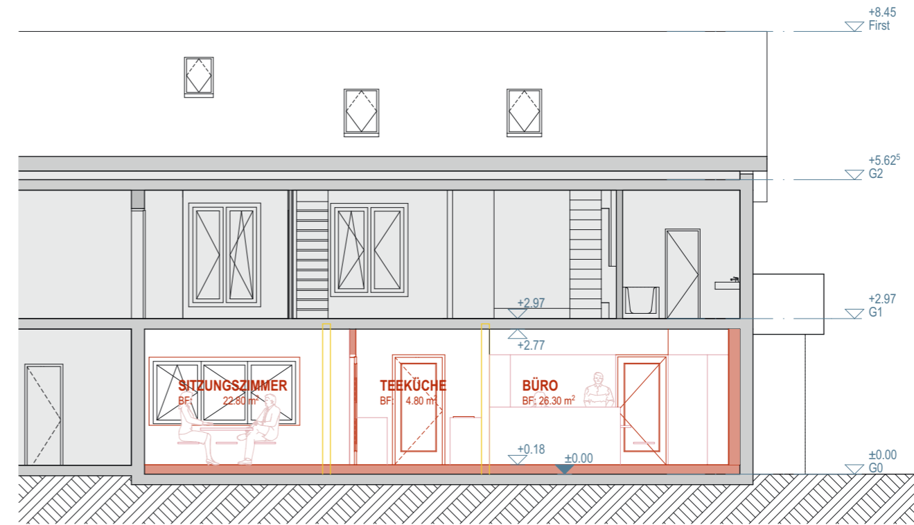
S/02 Längsschnitt
