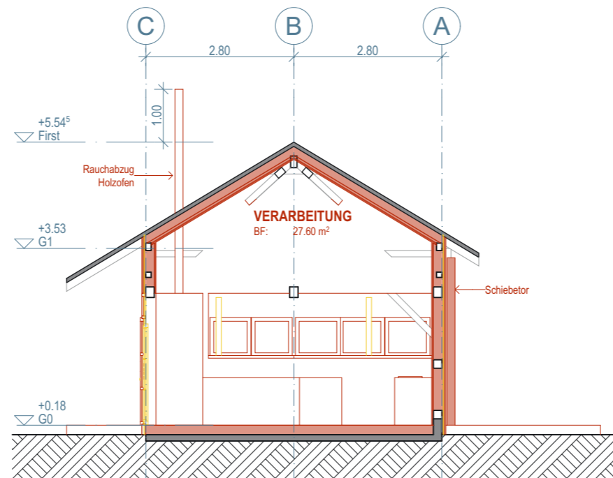
S/06 Querschnitt
