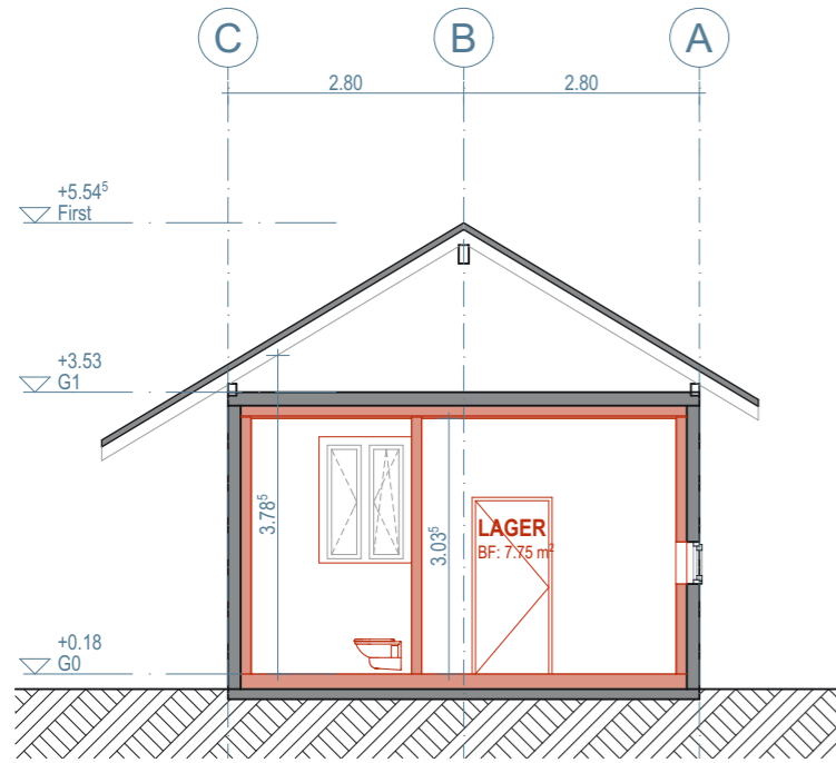
S/02 Querschnitt
