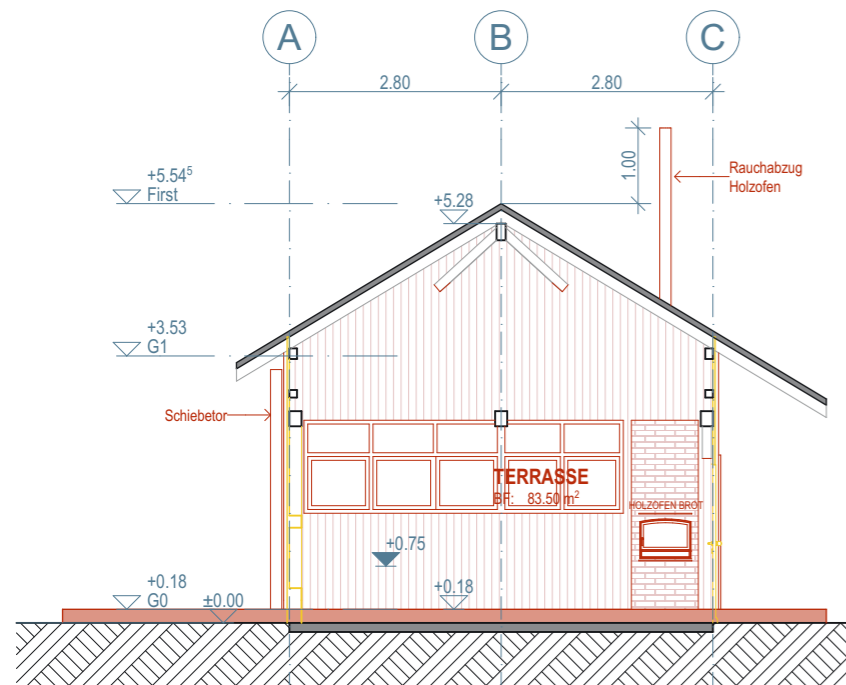
S/05 Querschnitt
