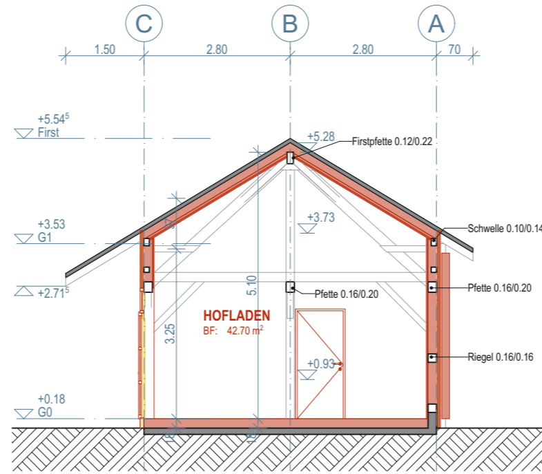
S/03 Querschnitt
