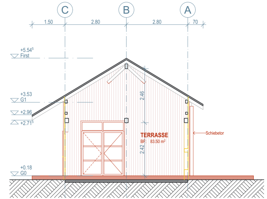
S/04 Querschnitt
