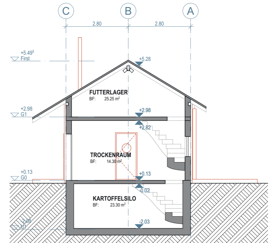
S/07 Querschnitt
